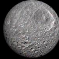
Mimas
