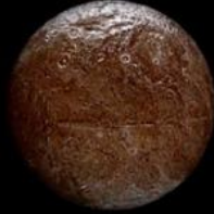
Iapetus
